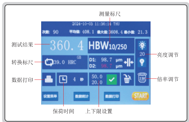
布氏测试界面
