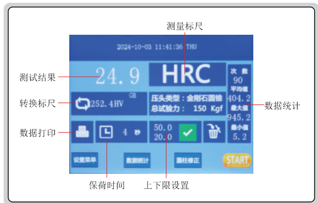
洛氏测试界面
